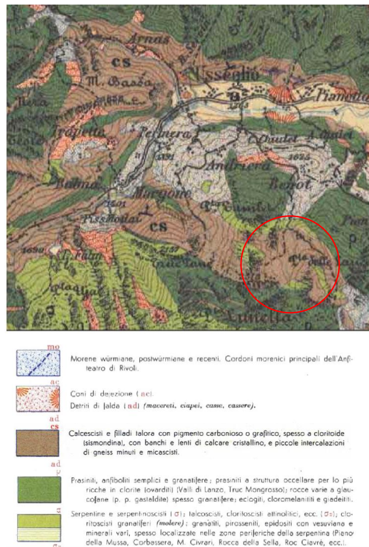
Figura 4. Schema geologico generale (Carta Geologica d'Italia alla scala 1:100.000)
