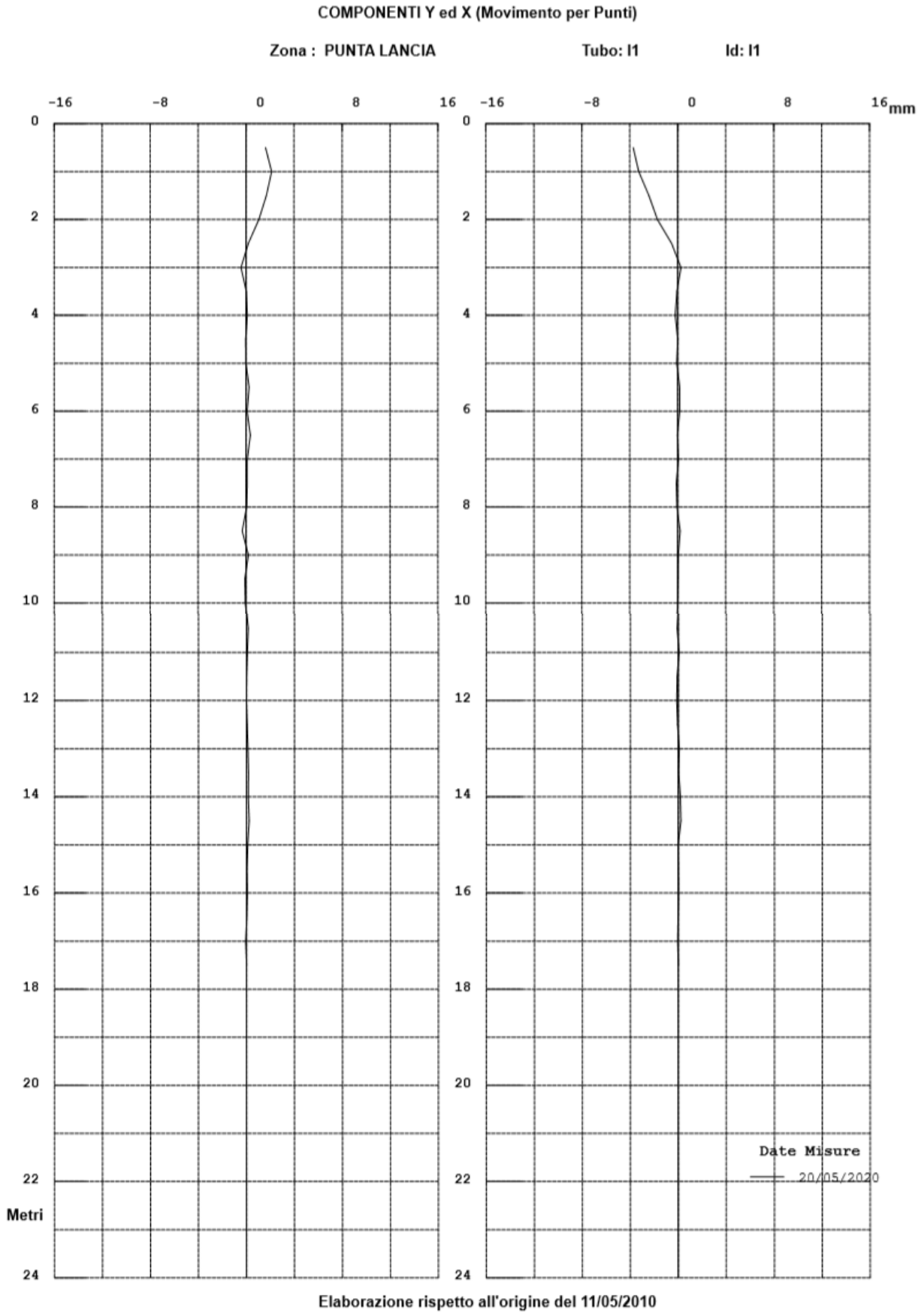
Figura 21. Spostamenti differenziali locali
