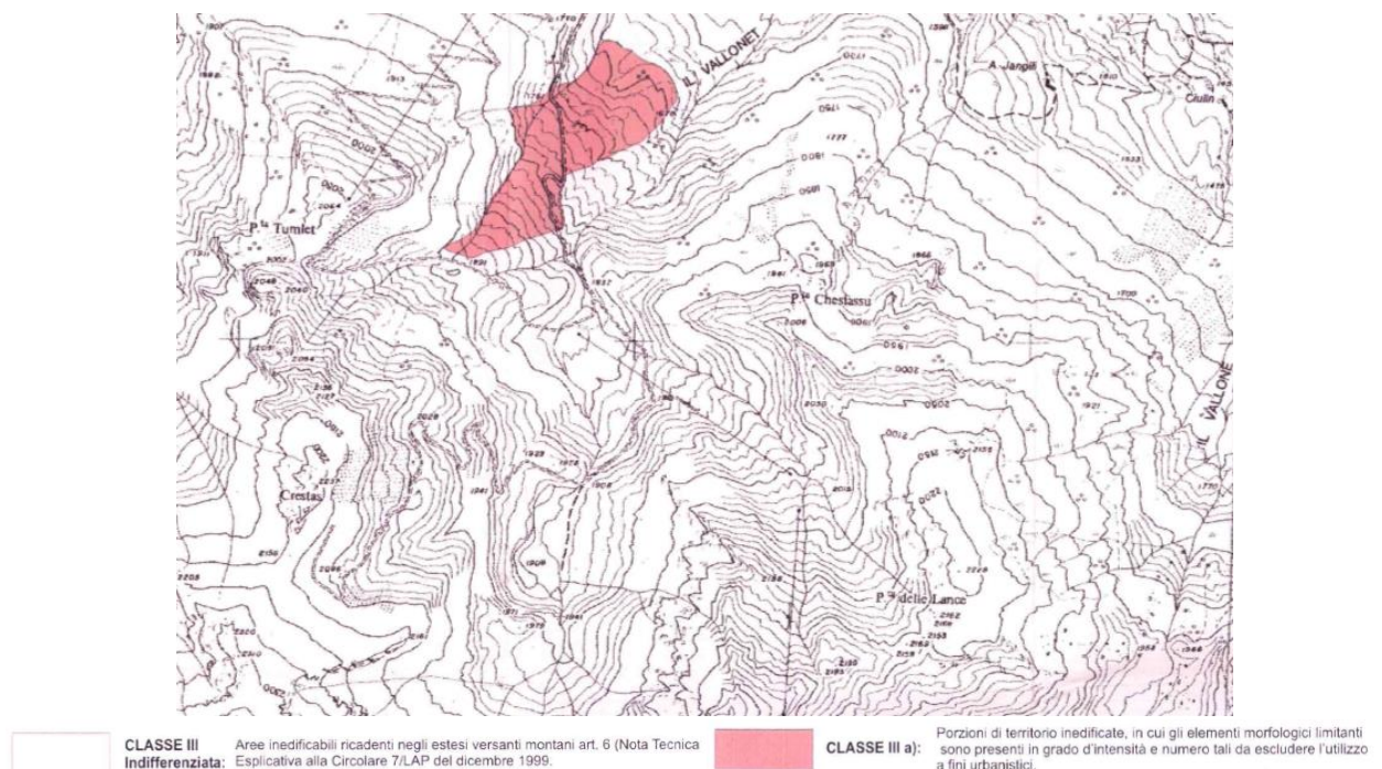
Figura 1. Carta della pericolosità geomorfologica (PRGC)
