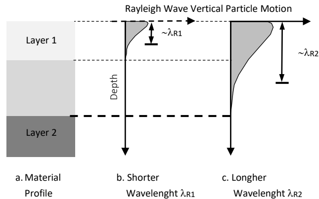
Figura 8. Profondità investigata dalle onde di Rayleigh in funzione della lunghezza d'onda, dalla velocità delle onde di taglio Vs e dalla frequenza (Stokoe e Santamarina, 2000).
