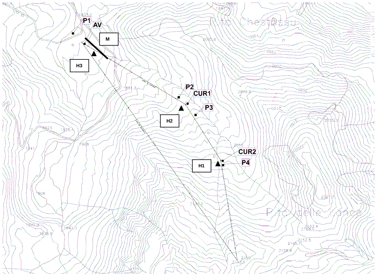
Figura 7. Ubicazione dei sondaggi AV, CUR1 e CUR2, dei pozzetti geognostici (P) e dei rilievi HVSR (H) e MASW (M).
