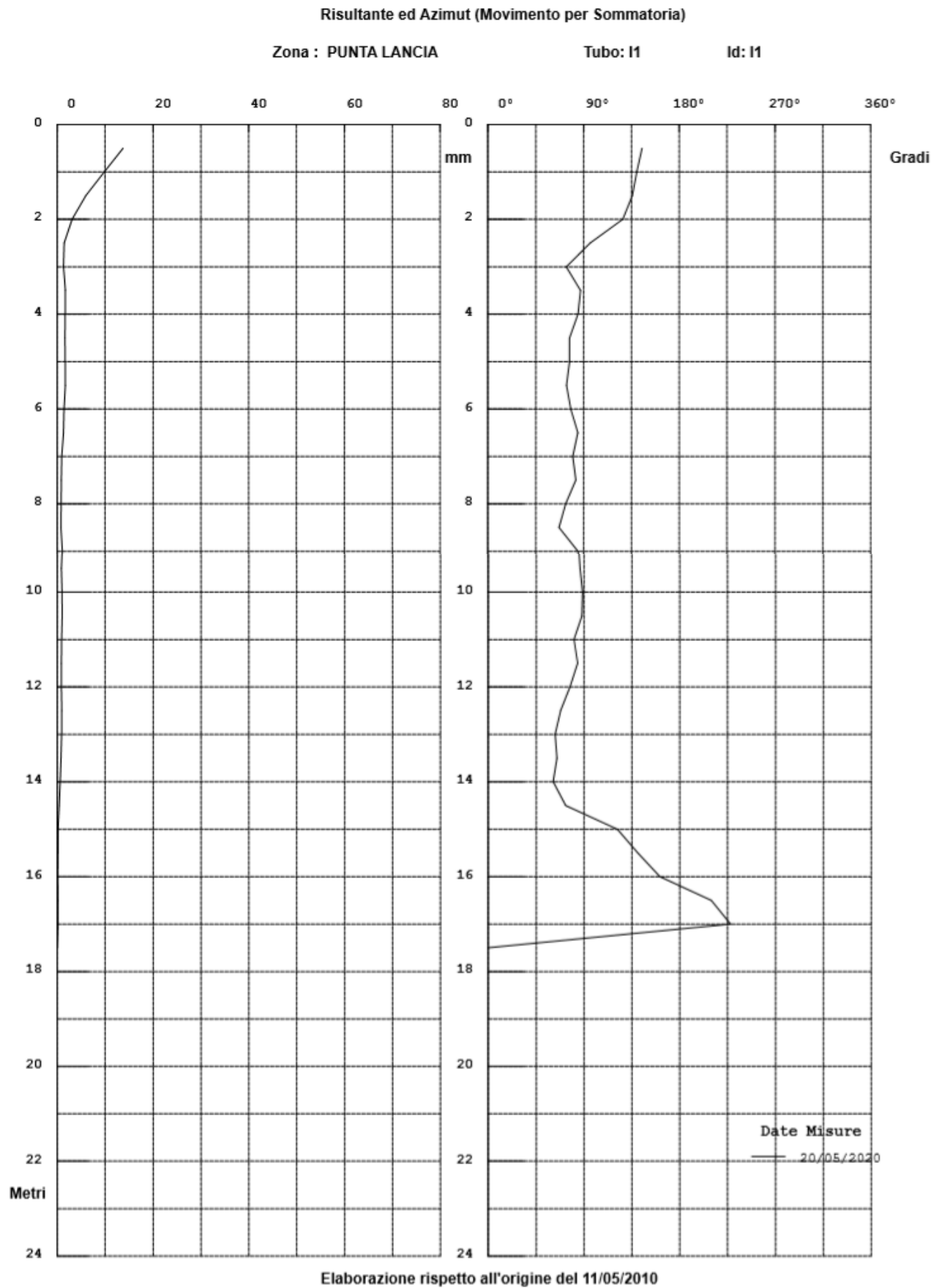
Figura 23. Spostamenti differenziali integrali
