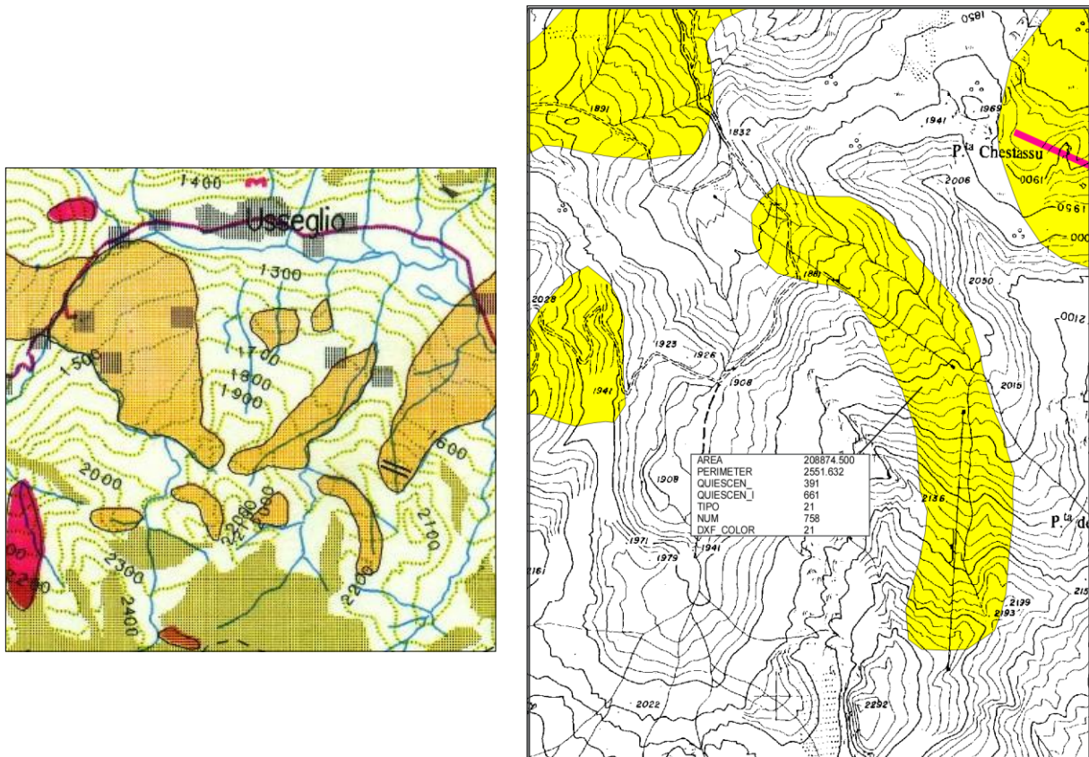
Figura 5. Stralcio Banca Dati Geologica ( www.regione.piemonte.it ) e Archivio RUPAR
