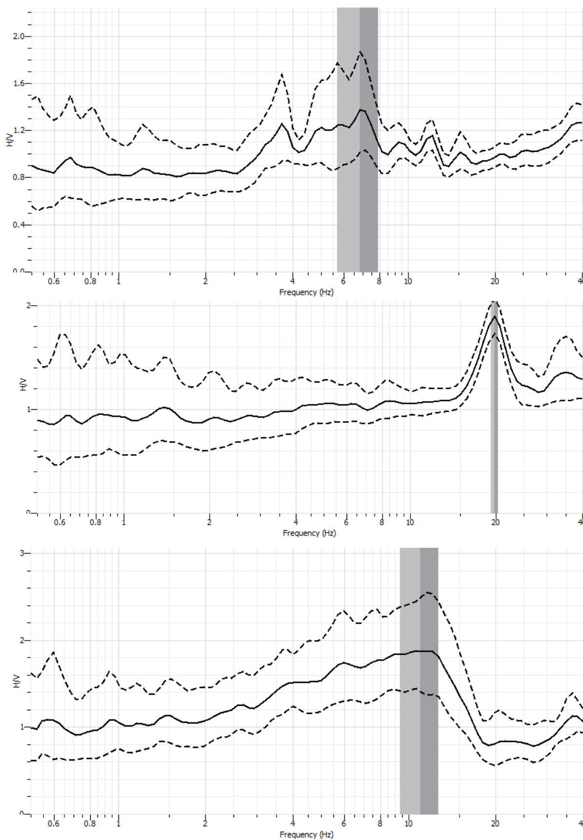
Figura 15. Sintesi dei risultati dei rilievi tromografici
