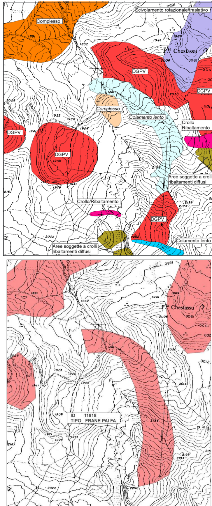
Figura 6. Stralcio Cartografia IFFI ( www.arpa.piemonte.it ), Stralcio Cartografia PAI/AiPO ( www.ai-po.it )
