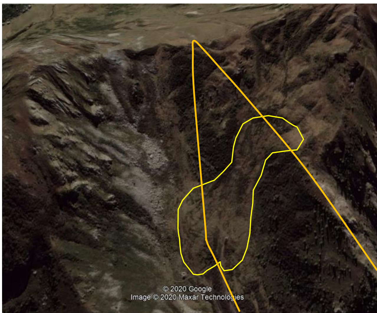
Figura 17. Delimitazione fenomeno di dissesto (Base Google Earth)
