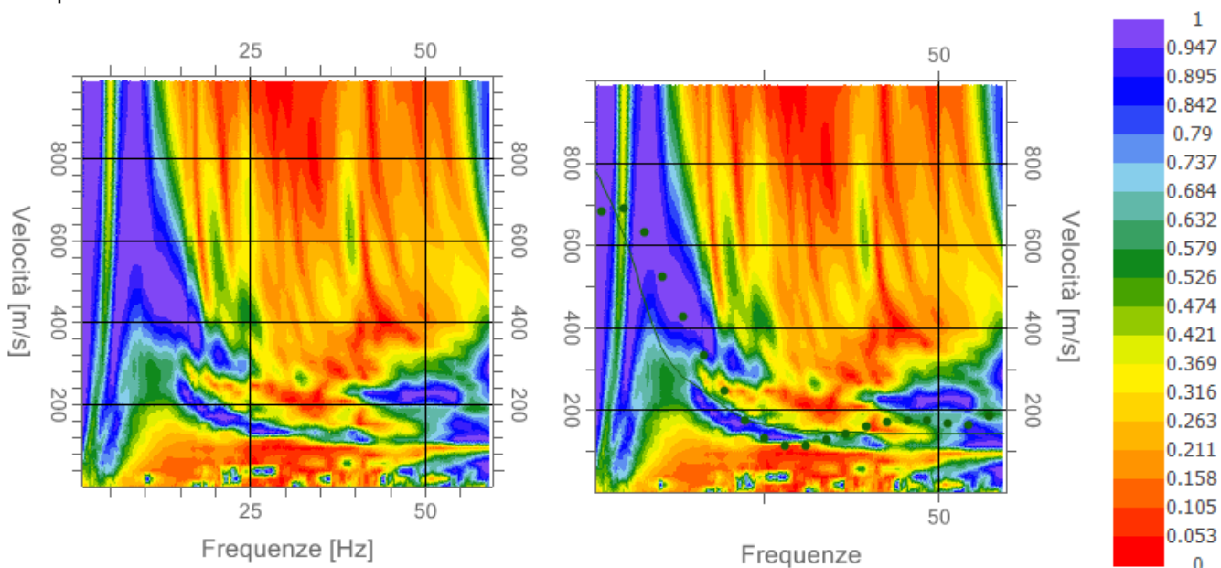
Figura 10. Spettro velocità di Fase / Frequenze ed inversione della curva
