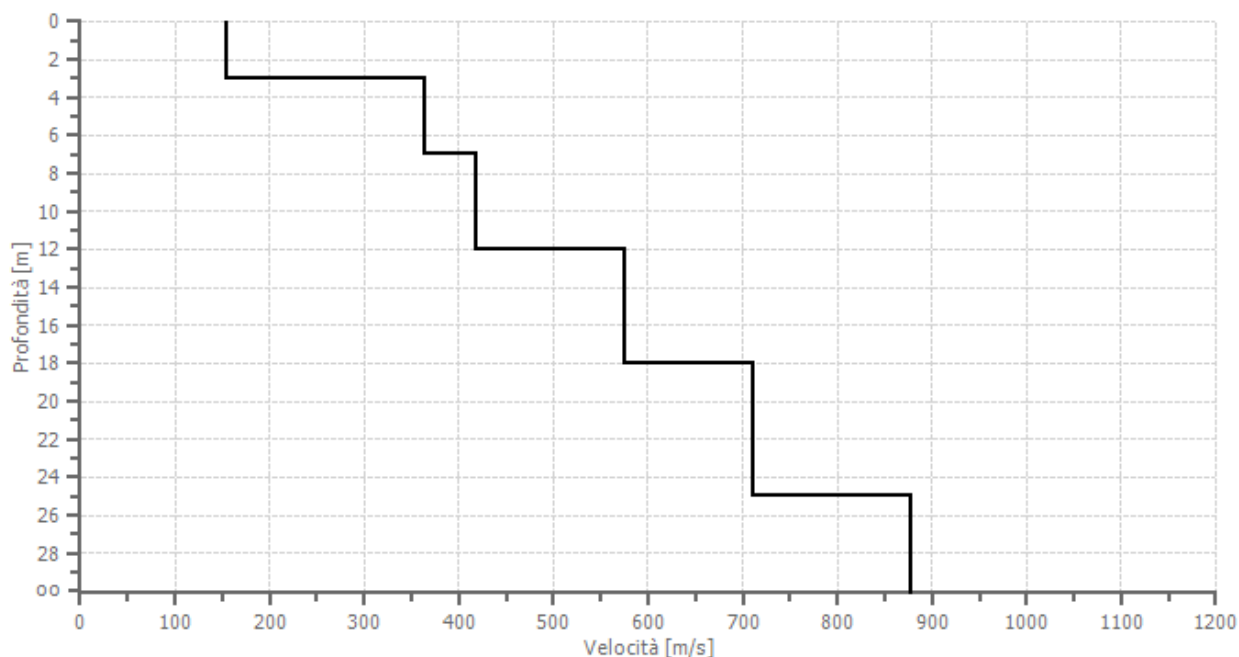
Figura 11. Profilo stratigrafico delle V_s
