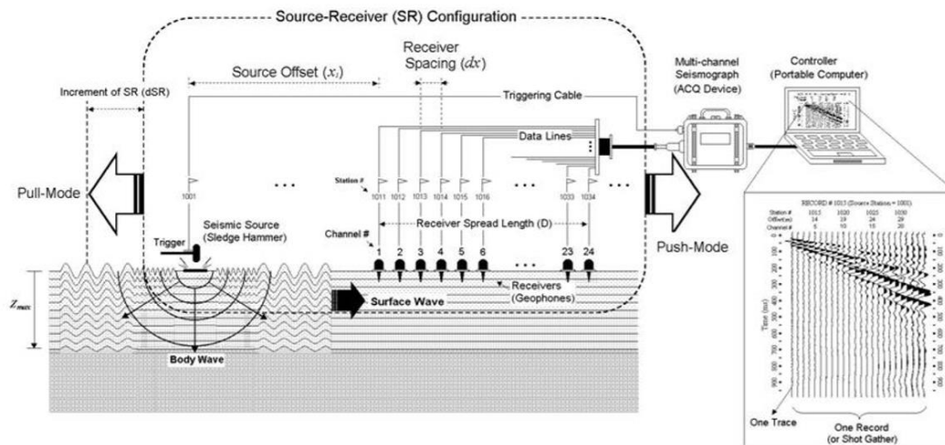
Figura 9. Schema tipo prospezione sismica MASW attiva
