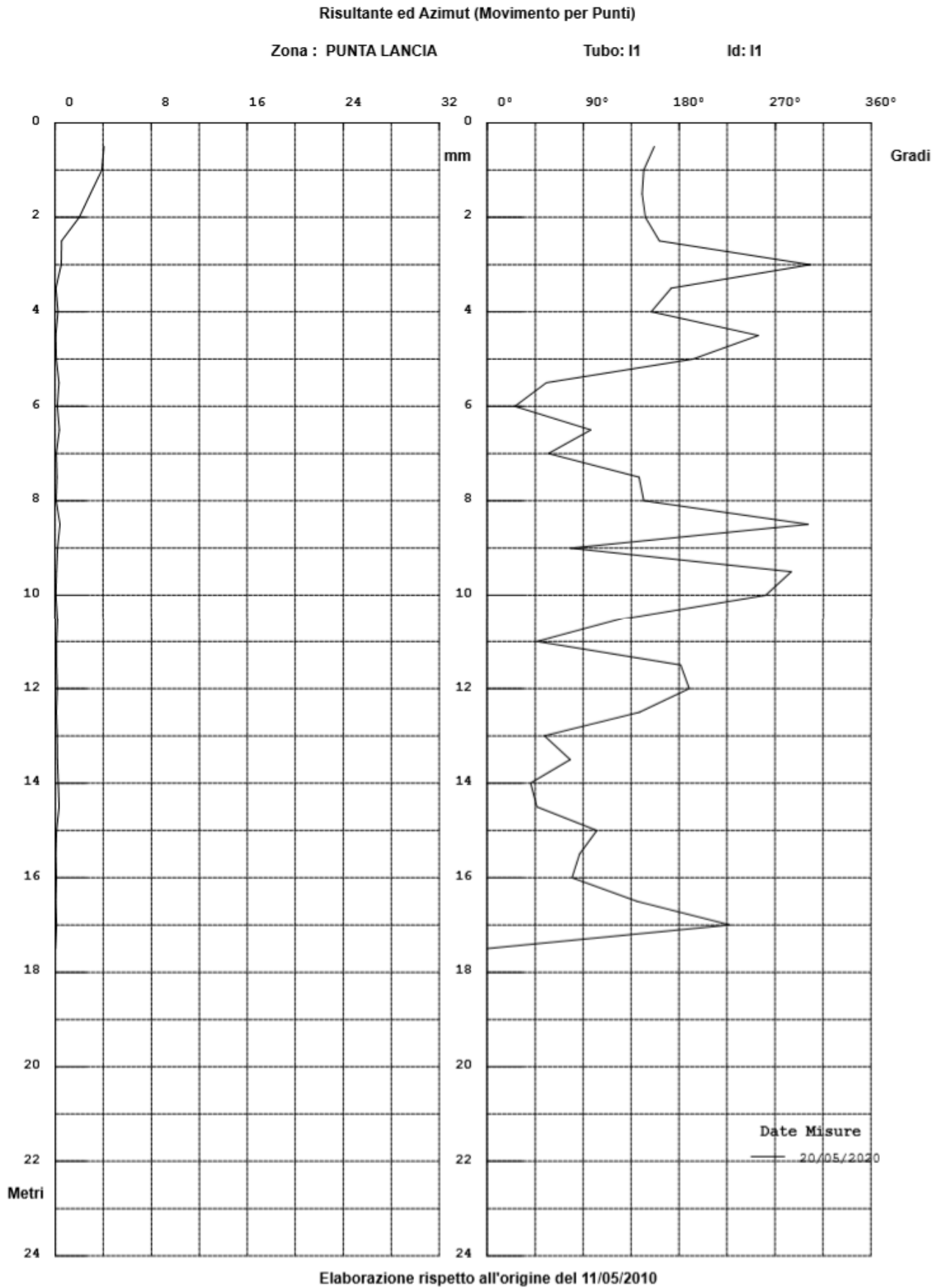
Figura 22. Spostamenti differenziali locali risultante
